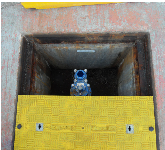
בעבר היה צורך בהסרת שני מכסי הפלדה הכבדים מאוד לגישה לשסתום הניתוק לאספקת מי שתייה. כעת יש צורך רק בהרמה של מכסה שוחה אחד של Fibrelite.
