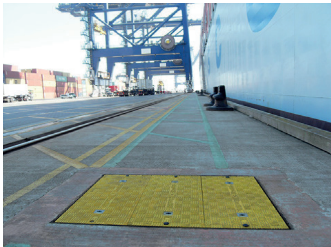
Lekkie pokrywy kanałowe w klasie obciążenia 90 ton w miejscu instalacji na nabrzeżu
