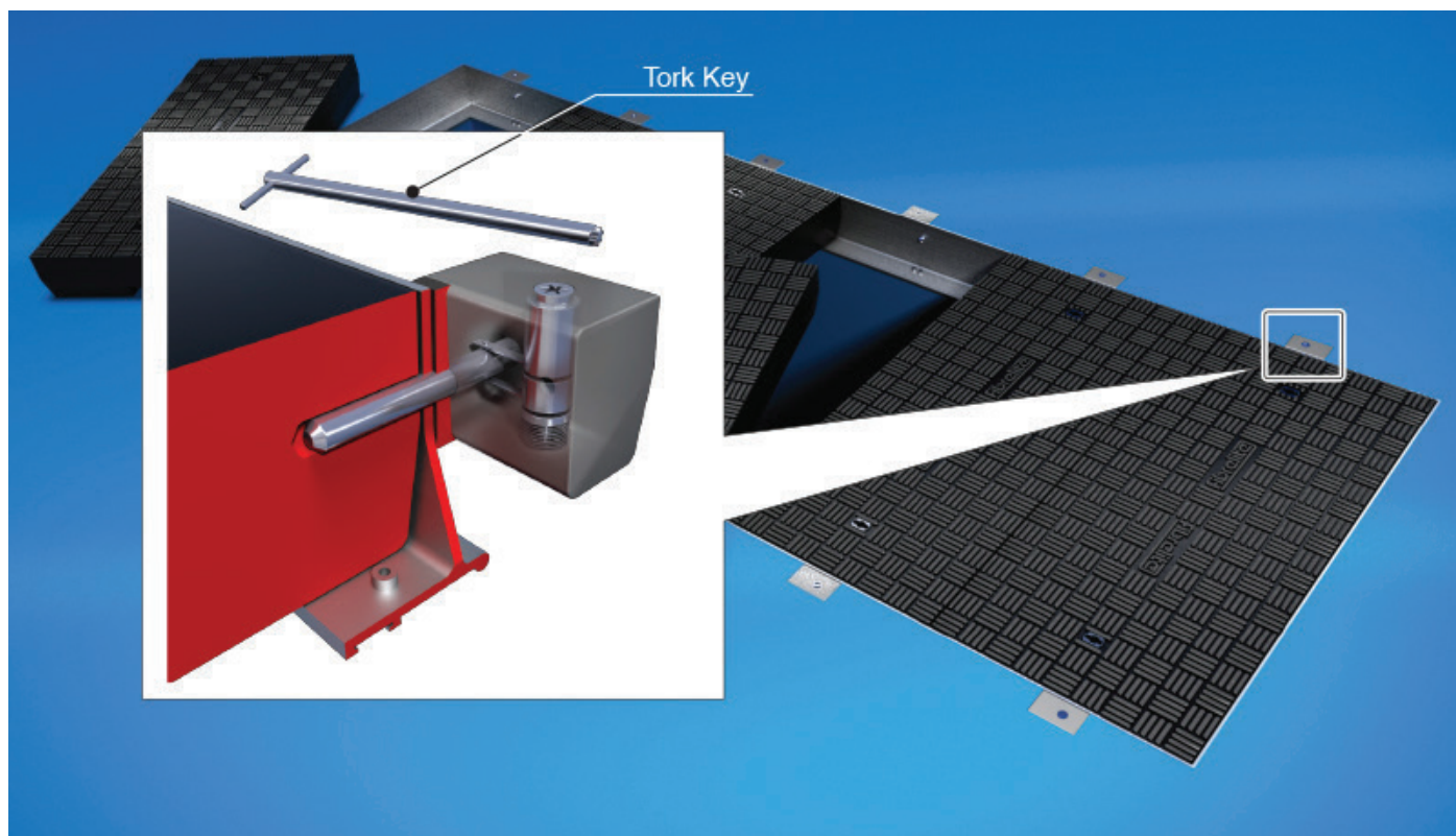
Bezobsługowe i niezmechanizowane: Fibrelite FM45 składane panele do wykopów
